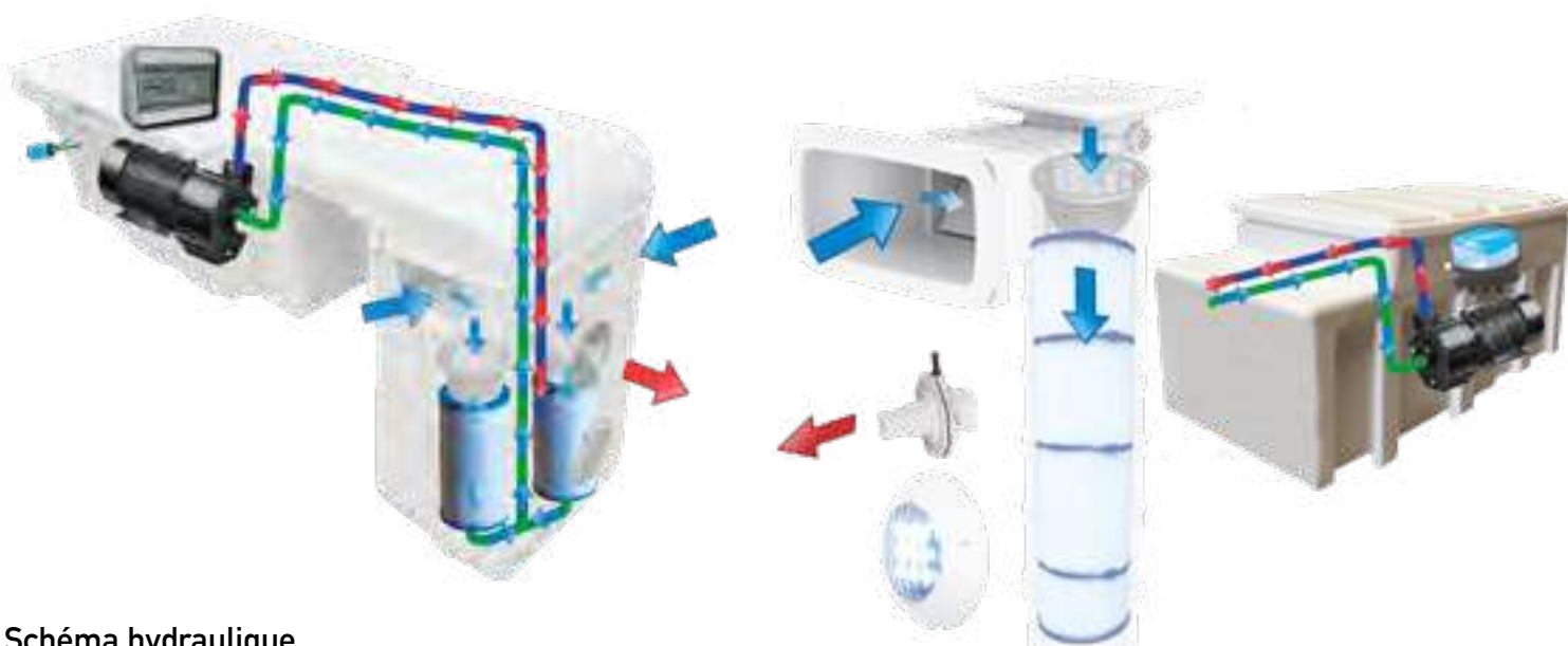
Schéma hydraulique de la paroi filtrante (standard hors options)
